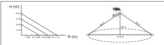
Fig. 11: Installazione - Raggiungere
